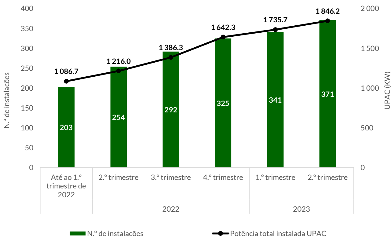
Gráfico 50. Número de instalações e potência instalada de UPAC, em Vouzela, até ao 2º trimestre de 2023
